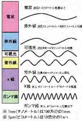
図：さまざまな電磁波と波長の関係
